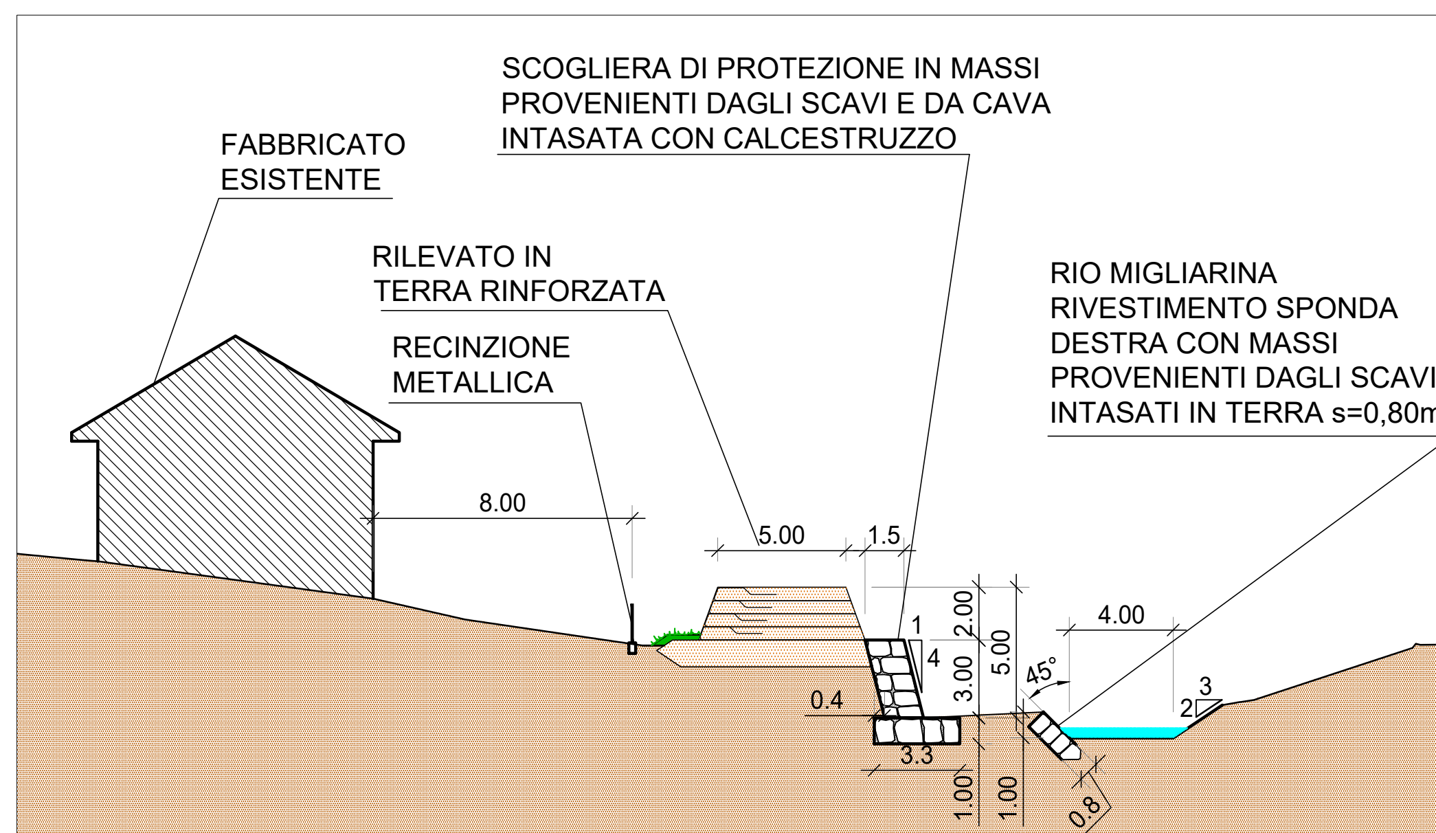
SEZIONE TIPO A - SC. 1:200
