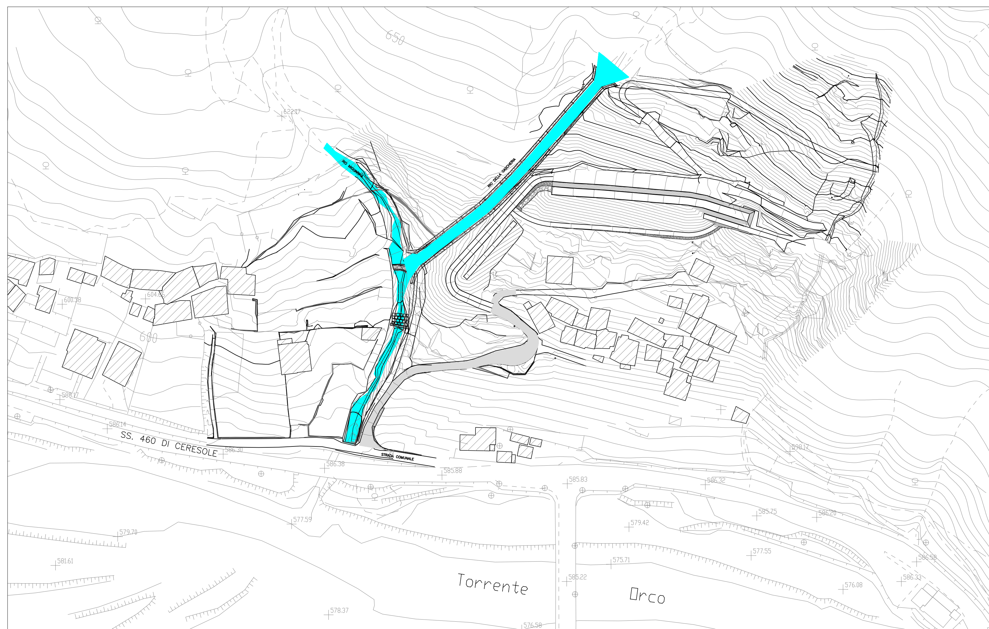
PLANIMETRIA DI PROGETTO sc. 1:500
