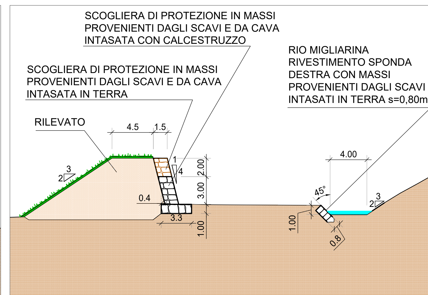
SEZIONE TIPO B - SC. 1:200
