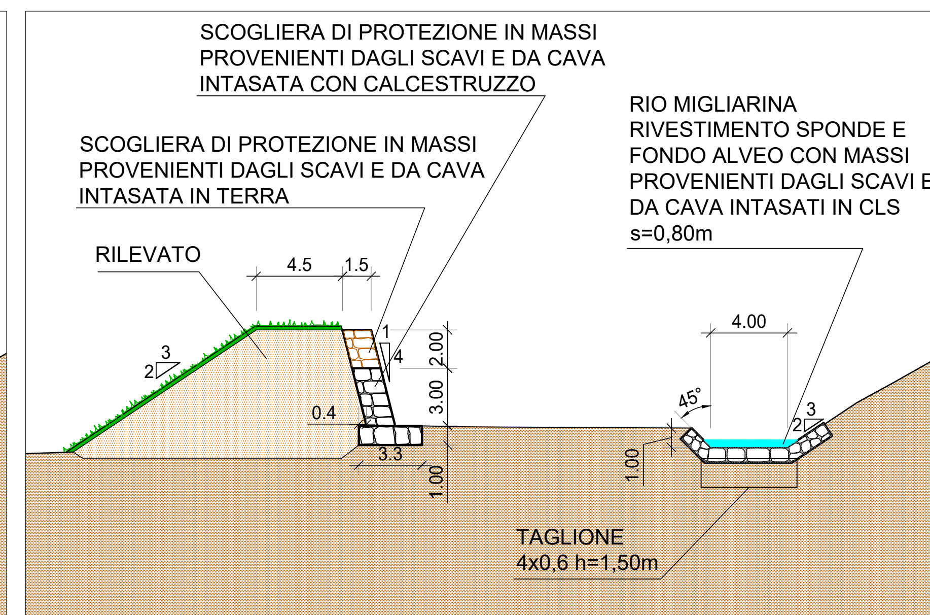
SEZIONE TIPO B (TRATTI DI ALVEO RIVESTITO) - SC. 1:200
